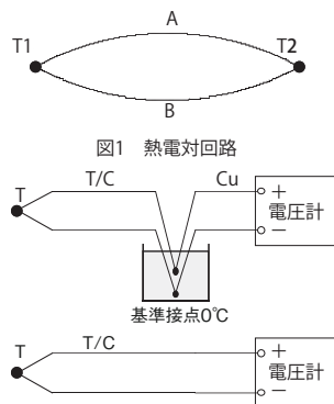
図2 熱電対と基準接点
