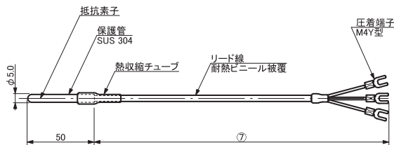
【型番: RLS-BLS-50UBHV-(L)】
