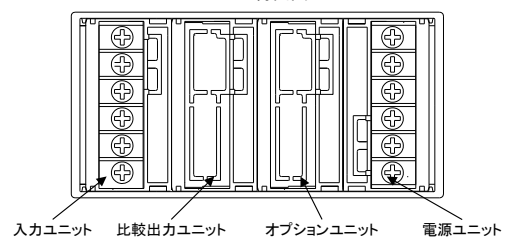
A6000背面図
