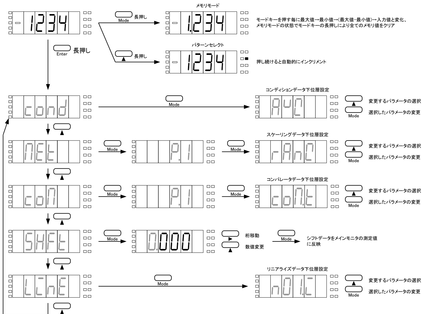
操作体系図
