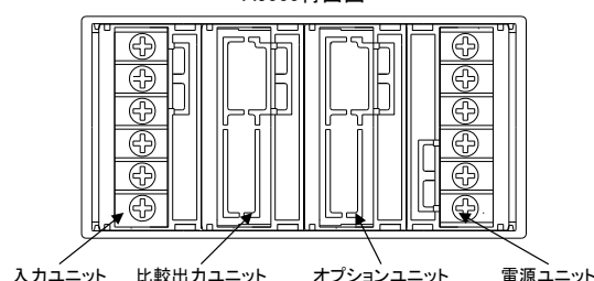
A6000背面図
