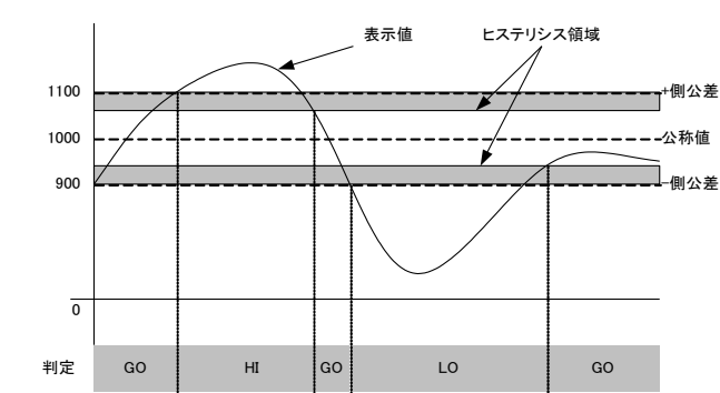
設定例2 交差判定モード
