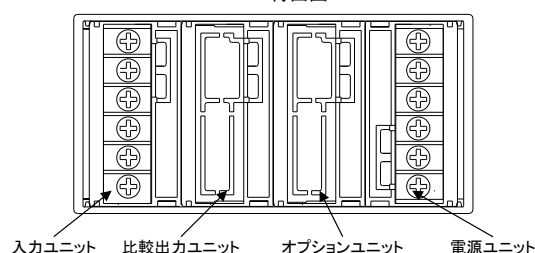
A6000背面図
