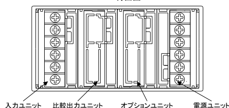
A6000背面図
