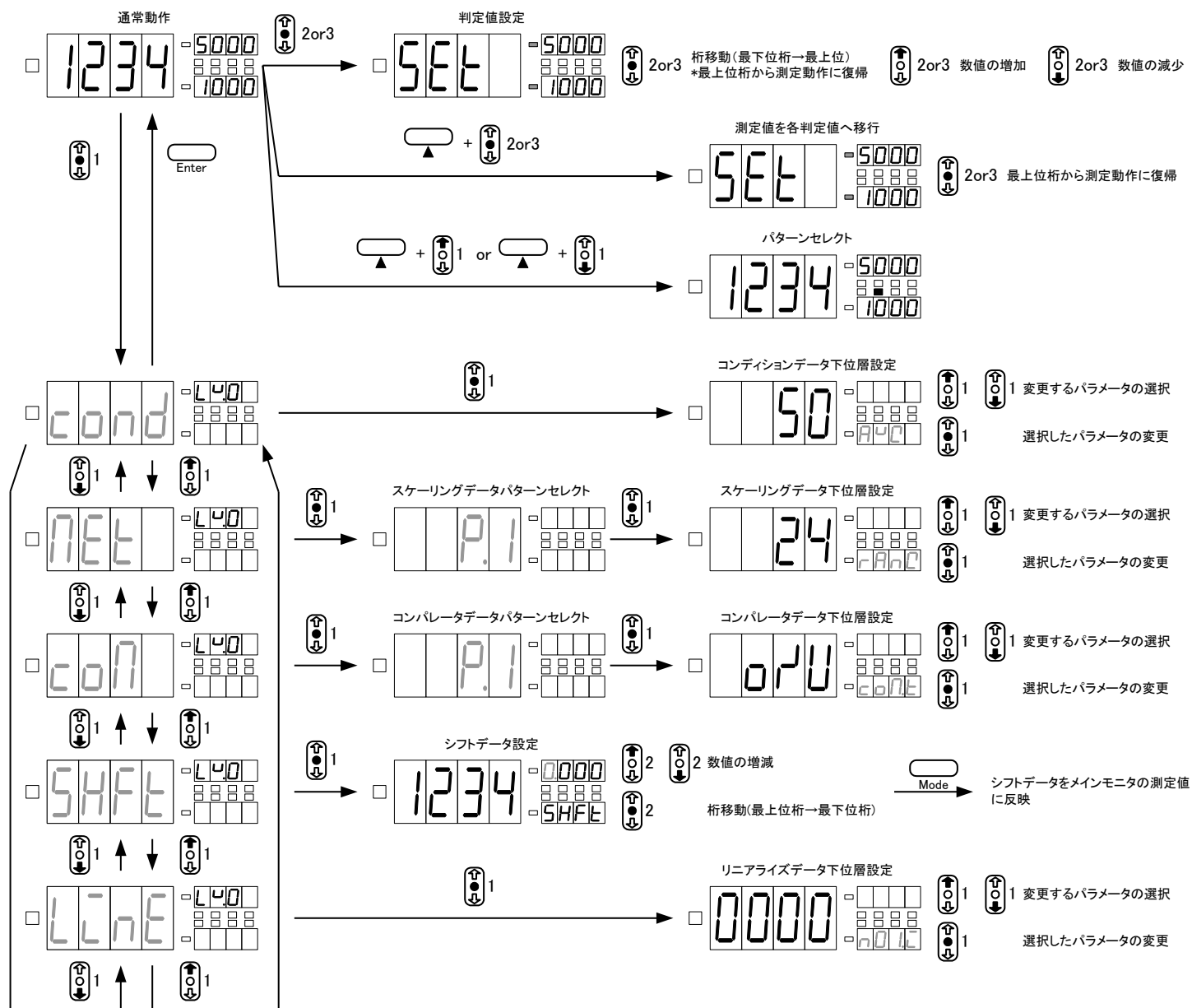
操作体系図
