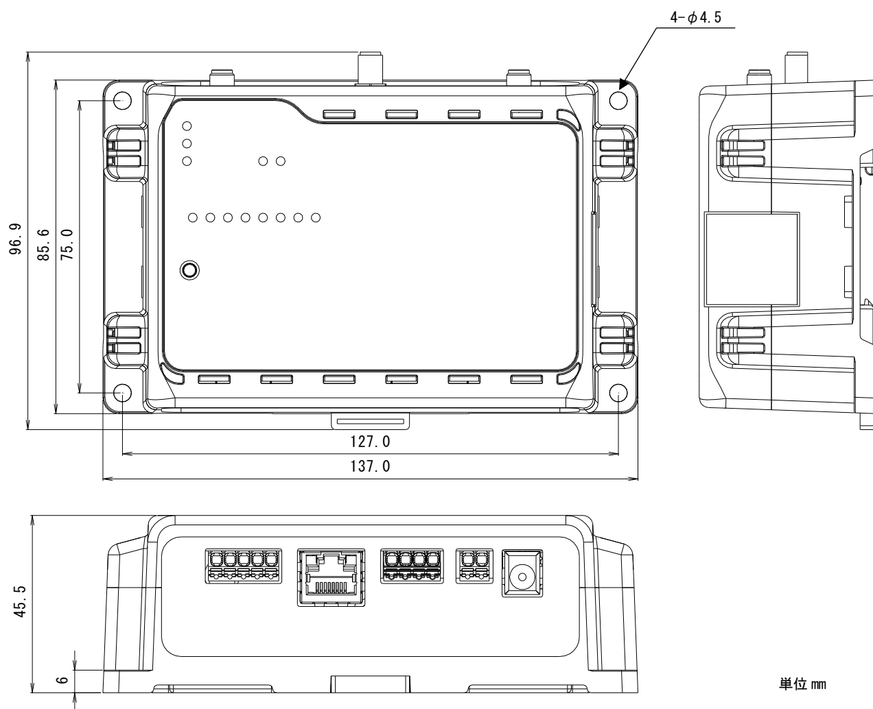
図 4-2 外観図
