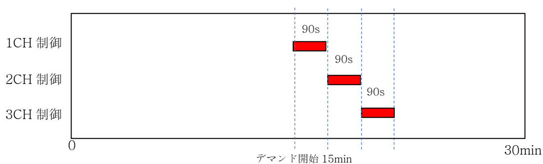
図 8-4 デマンド予測制御
