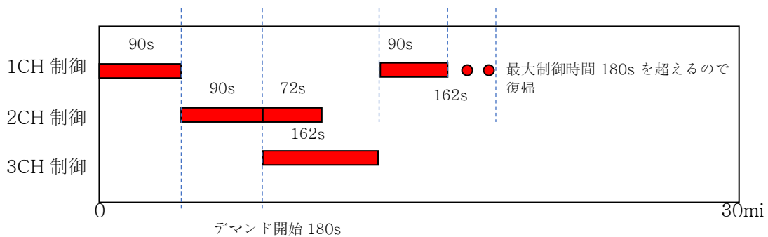
図 8-5 常時+デマンド予測制御
