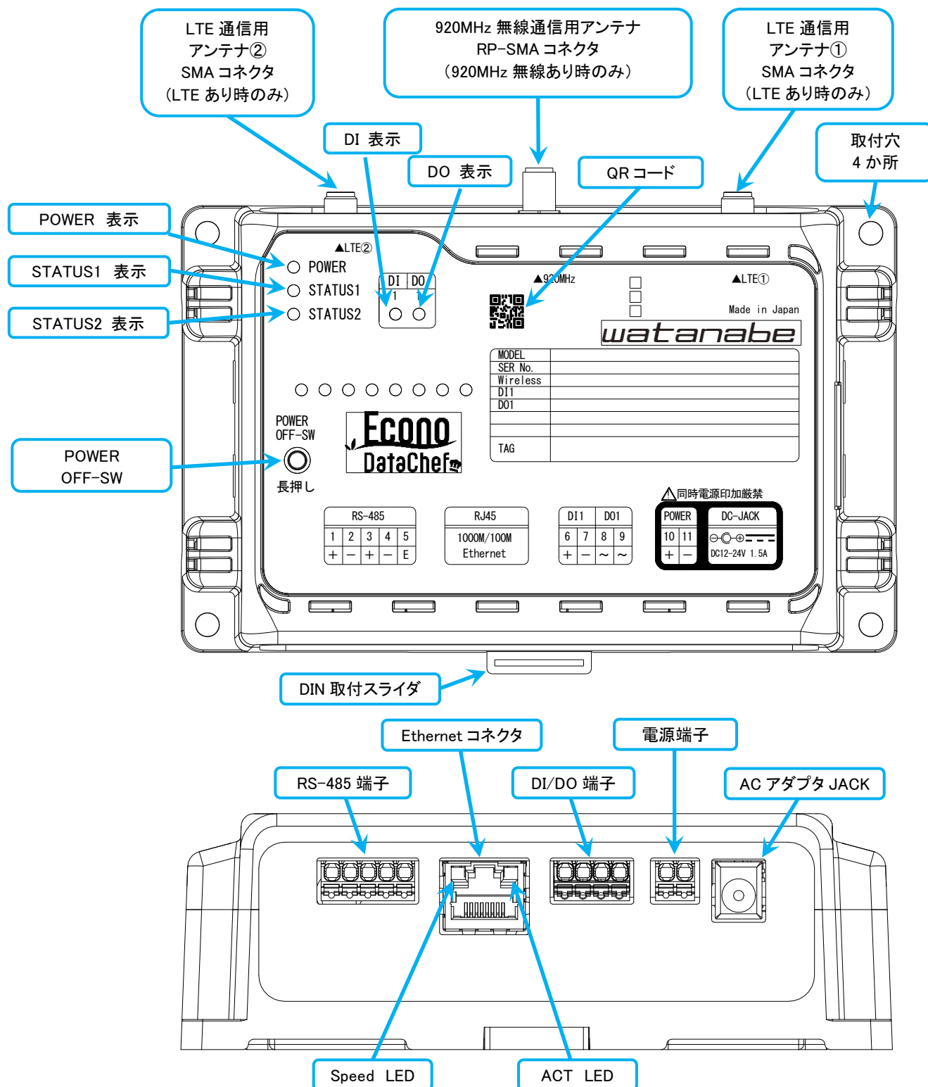
図 4-1 外観説明
