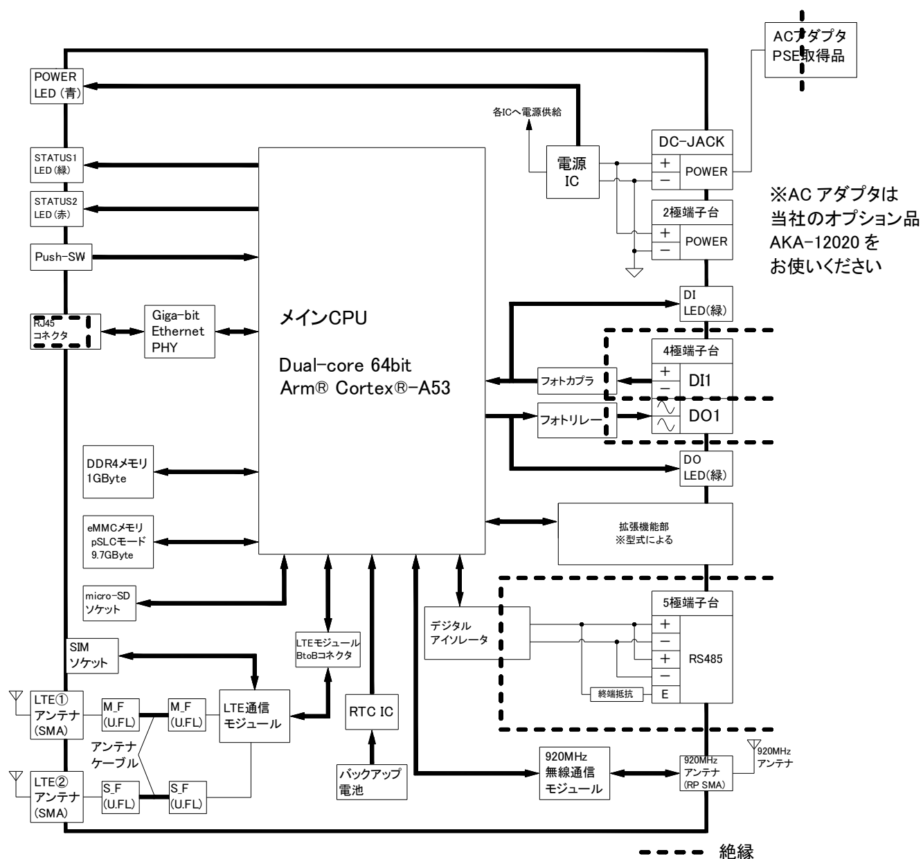
図 5-1 ブロック図
