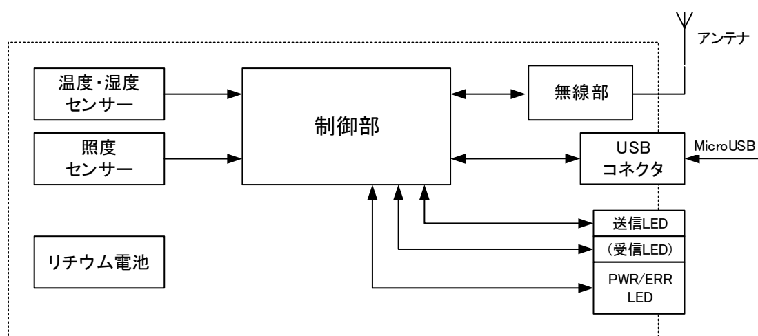
図 5 ブロック図
