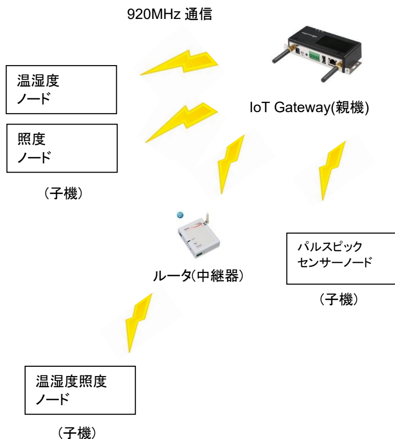
図 4 無線センサネットワーク構成例
