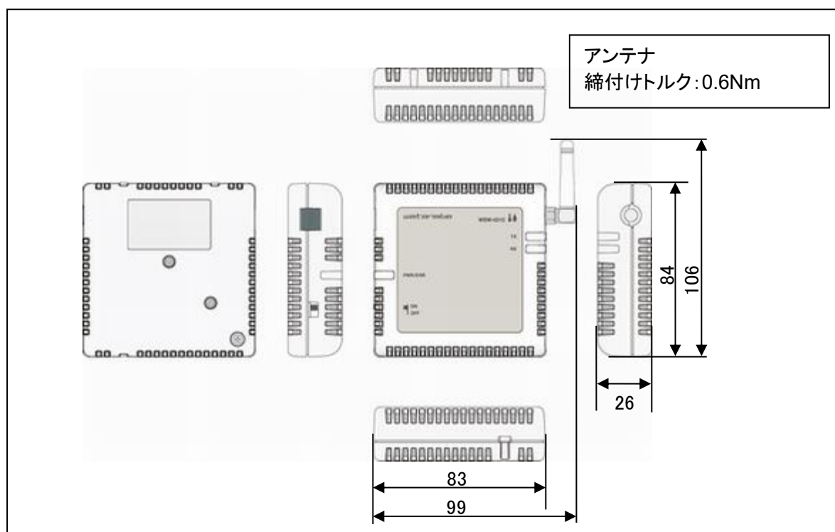
図 6 外形寸法図 (WSW-421C-1202)
