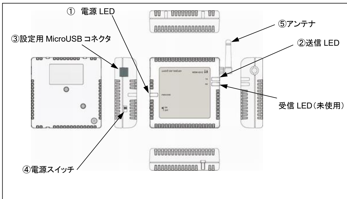
図 1 外観と各部の名称 (WSW-421C-1202)
