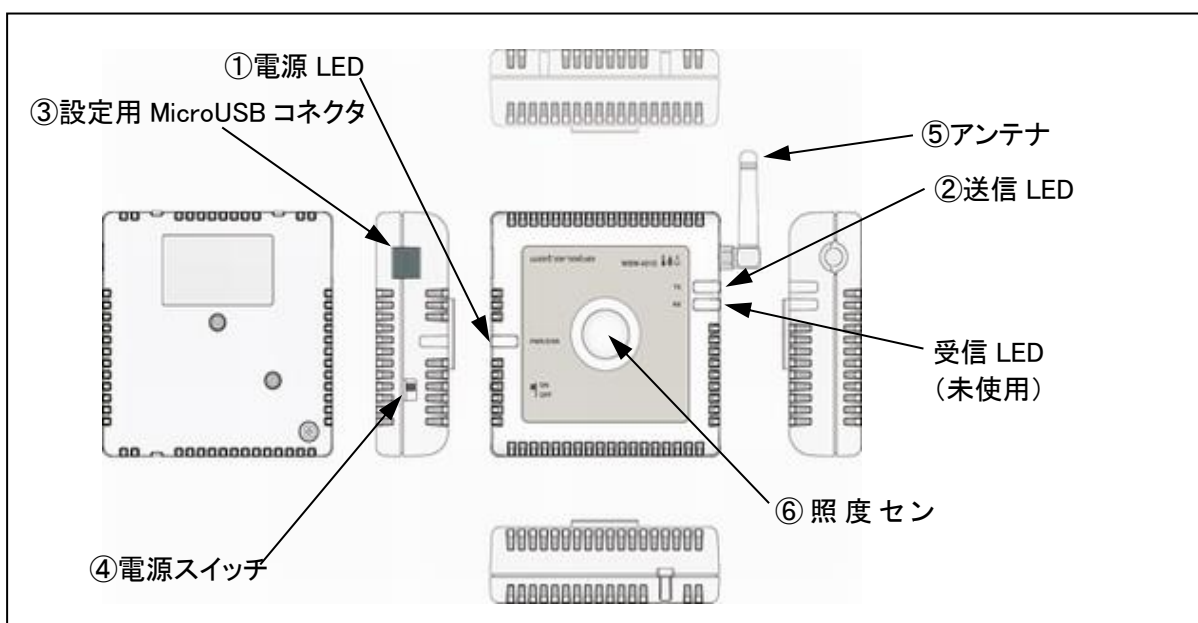
図 2 外観と各部の名称 (WSW-421C-1204)
