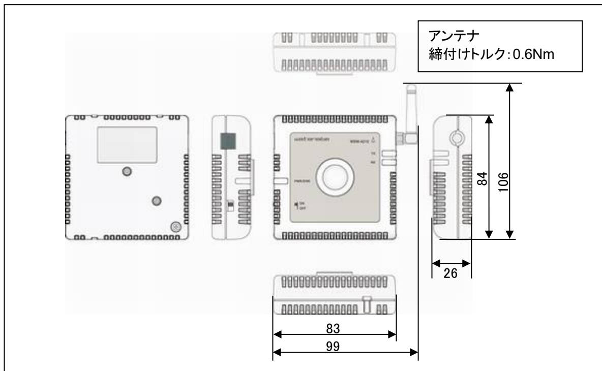
図 8 外形寸法図(WSW-421C-1205)
