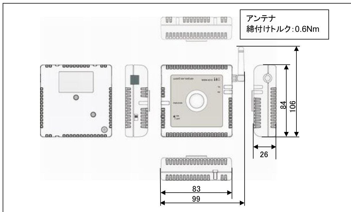
図 7 外形寸法図 (WSW-421C-1204)
