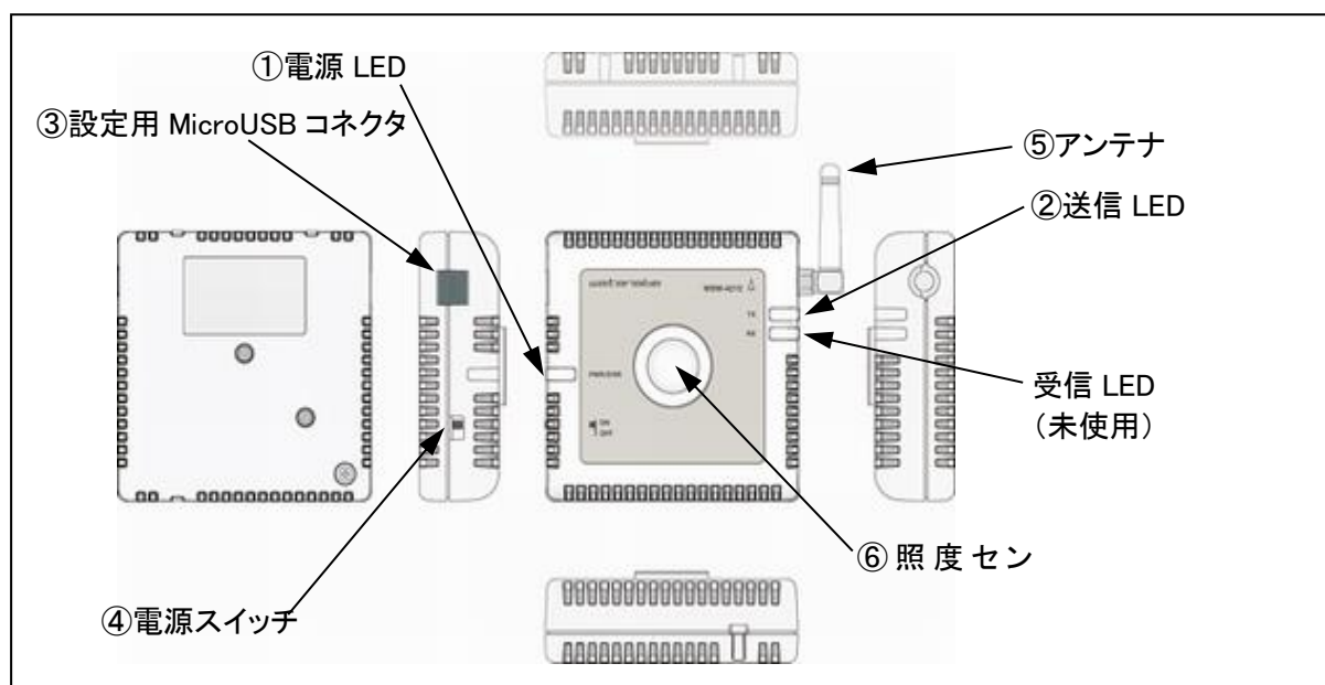
図 3 外観と各部の名称 (WSW-421C-1205)
