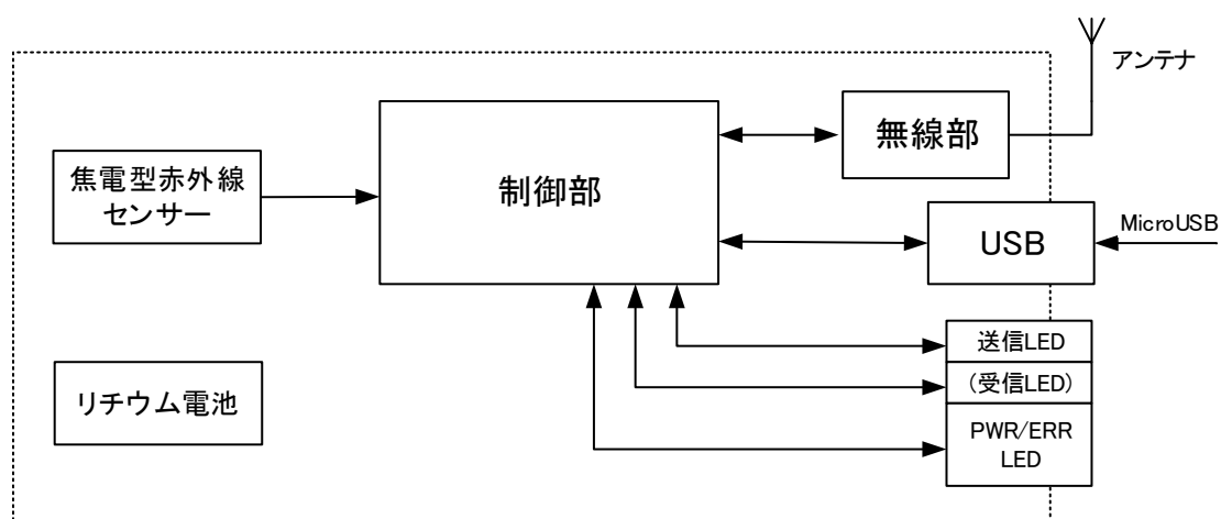
図 3 ブロック図
