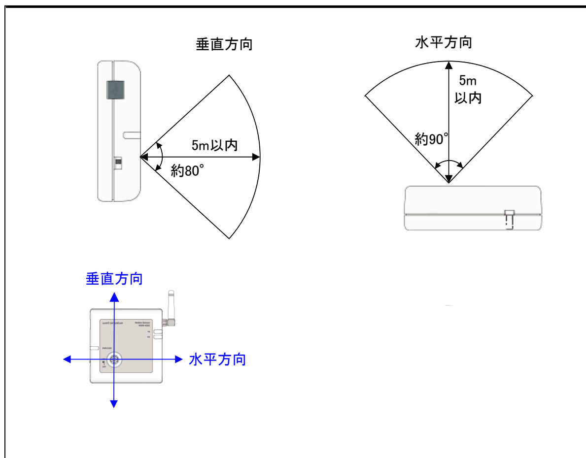
図 6 検出範囲
