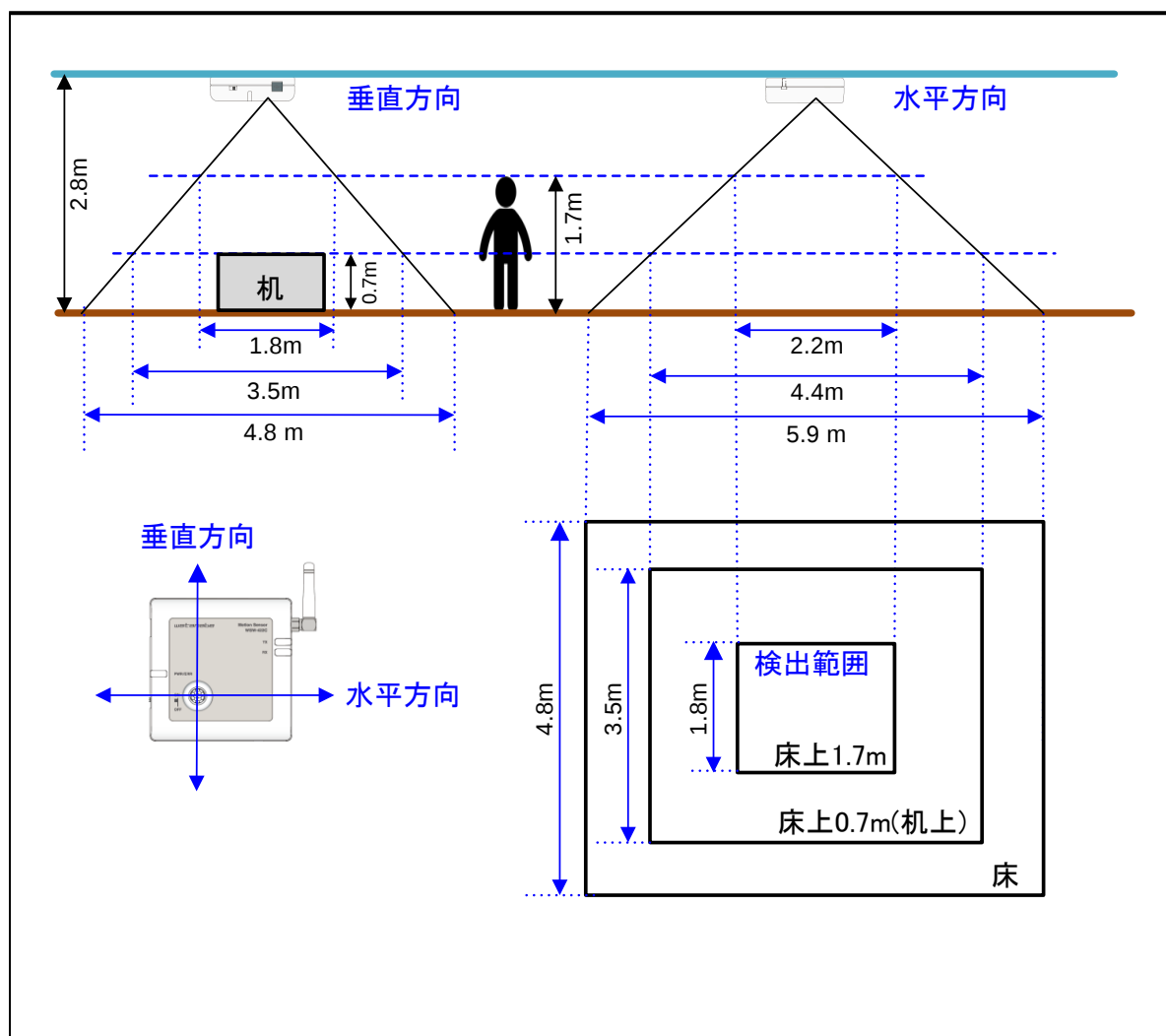
図 7 検出範囲例
