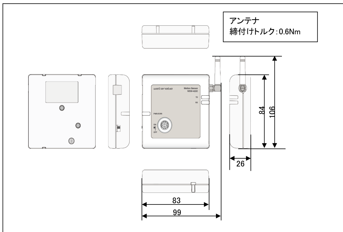
図 4 外形寸法図
