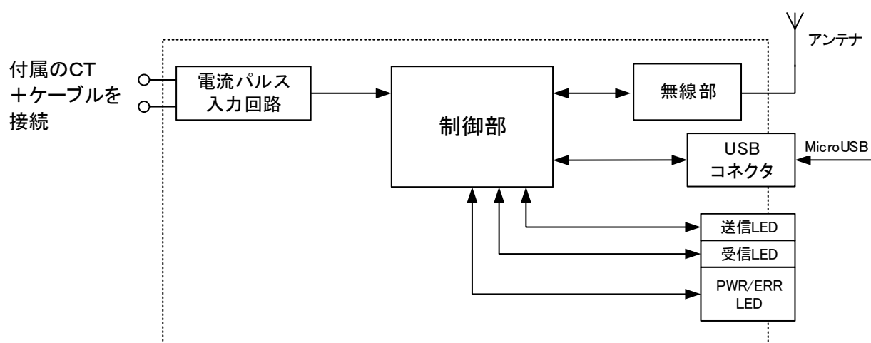
図 3 ブロック図
