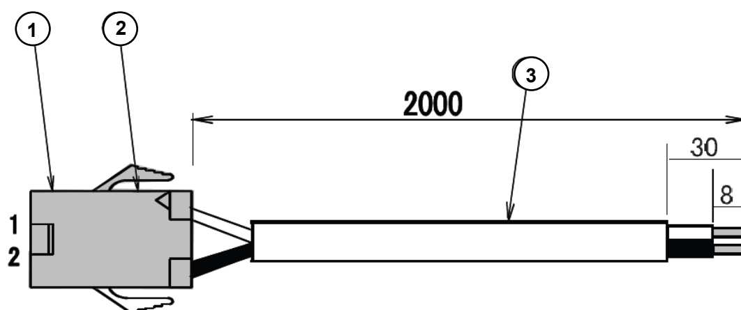
図 14 CT 接続ケーブル
