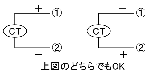
図 7 CT の極性
