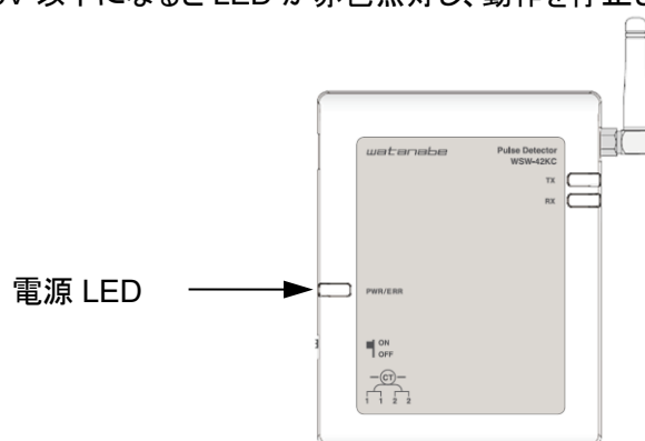
図 10 電池切れ表示
