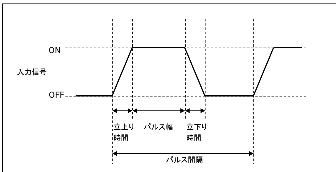
図 9 電流パルス波形
