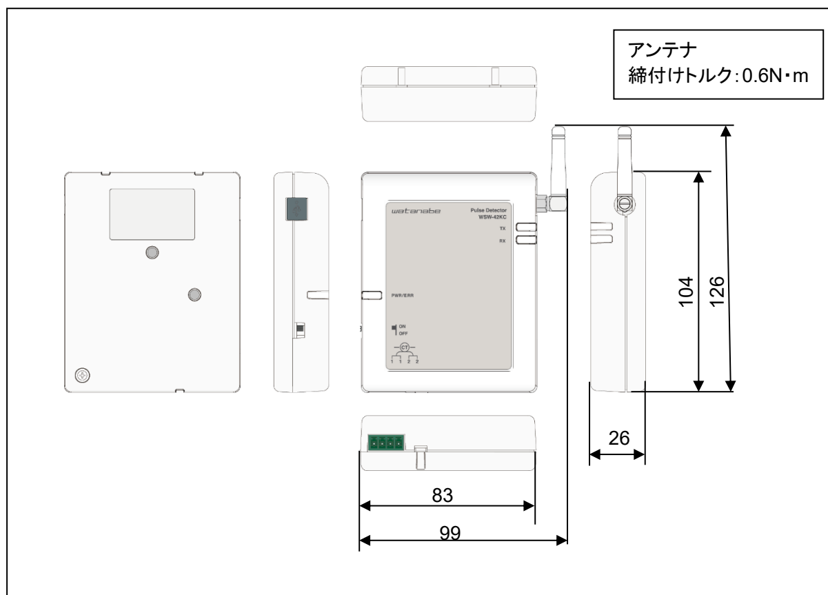
図 4 外形寸法図
