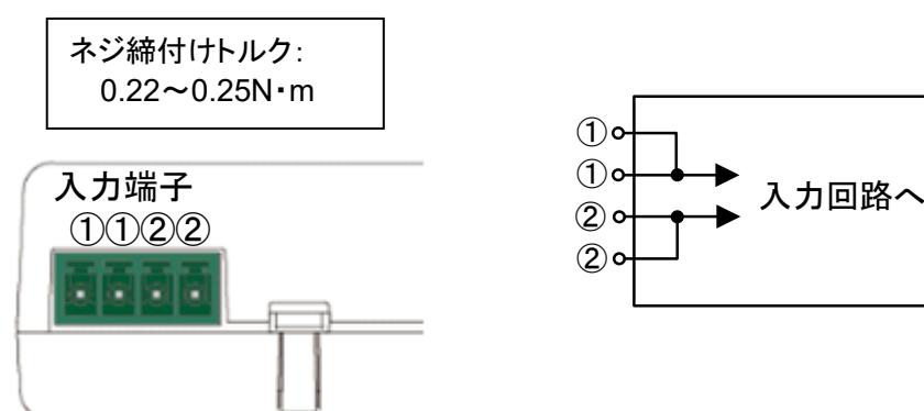
図 6 CT 接続用端子説明
