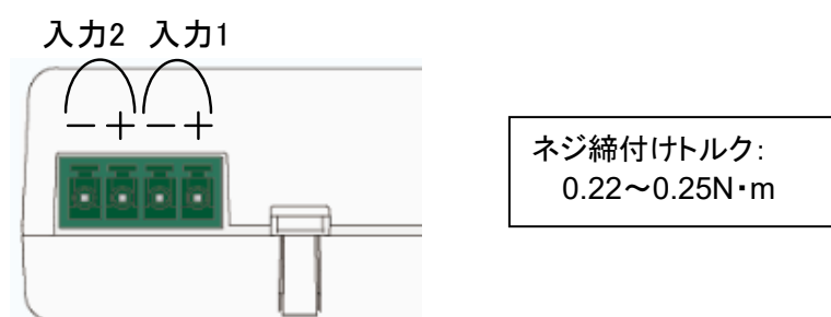
図 6 CT 接続用端子説明
