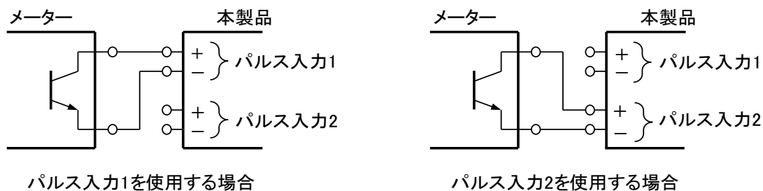
図 9 オープンコレクタ接続の場合
