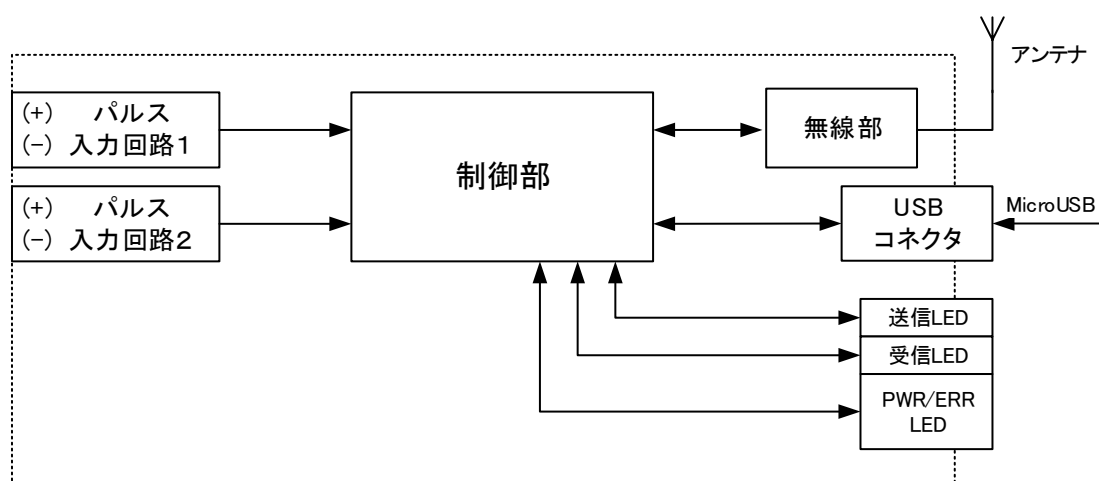
図 3 ブロック図
