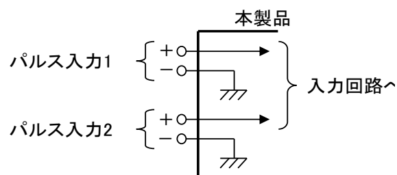
図 8 本製品のパルス入力端子
