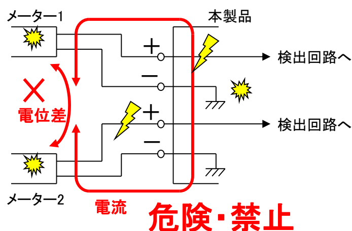
図 11 電位差のあるメータ2台の接続禁止
