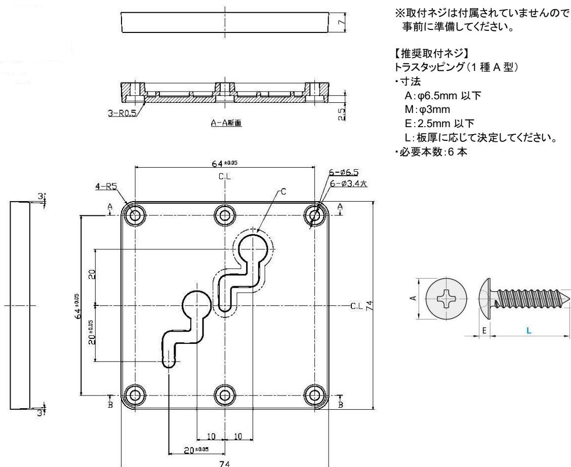
図 5 取付けプレートの外形寸法図
