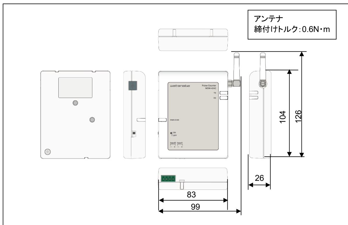
図 4 外形寸法図
