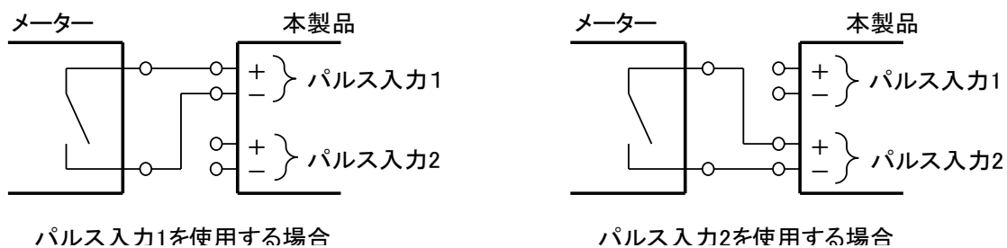
図 10 無電圧 a 接点接続の場合
