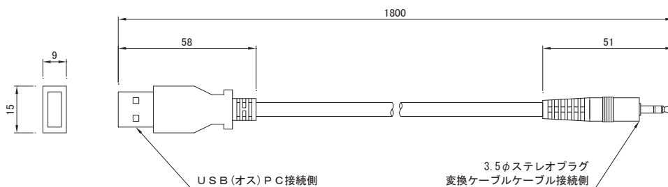
シリアルコンバータケーブル
