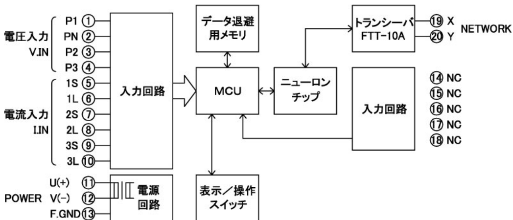
OWCD-PA34F 三相4線回路ブロック図
