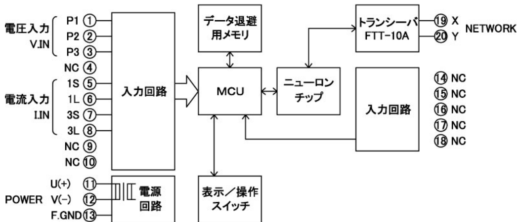
OWCD-PA13F/PA33F 単相3線／三相3線回路ブロック図
