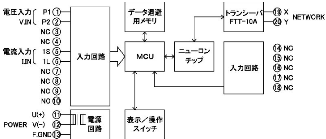
OWCD-PA12F 単相2線回路ブロック図
