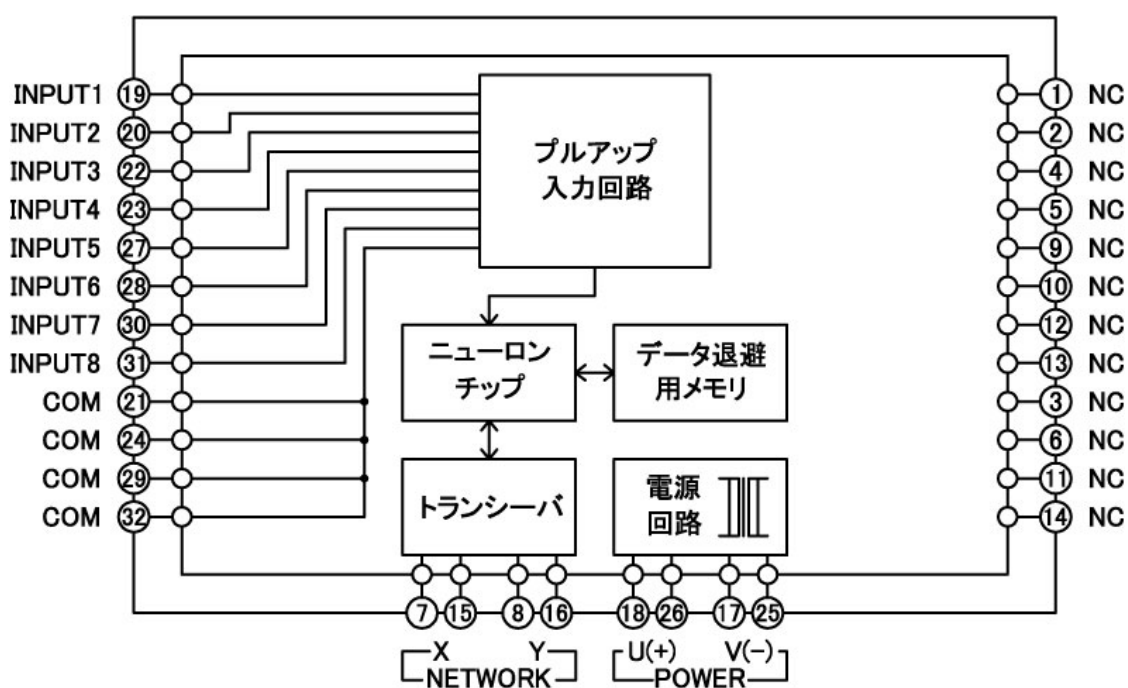
P I □ F回路ブロック図
