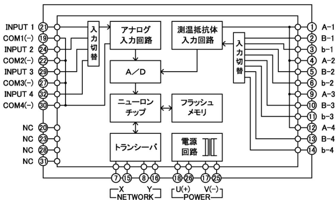
MA18F回路ブロック図
