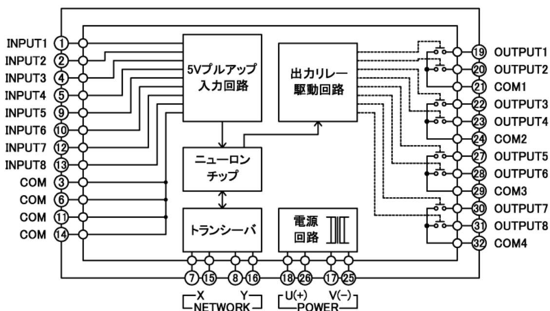
D I O 8 R F 回路ブロック図
