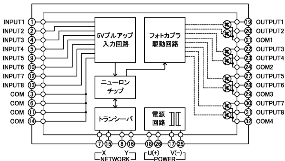
DI08T回路ブロック図
