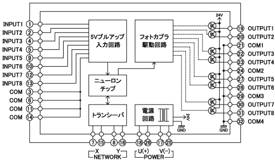
D I O 8 V F 回路ブロック図
