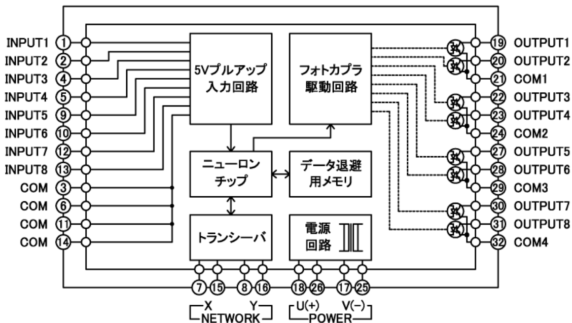
D I O 8 Y 回路ブロック図
