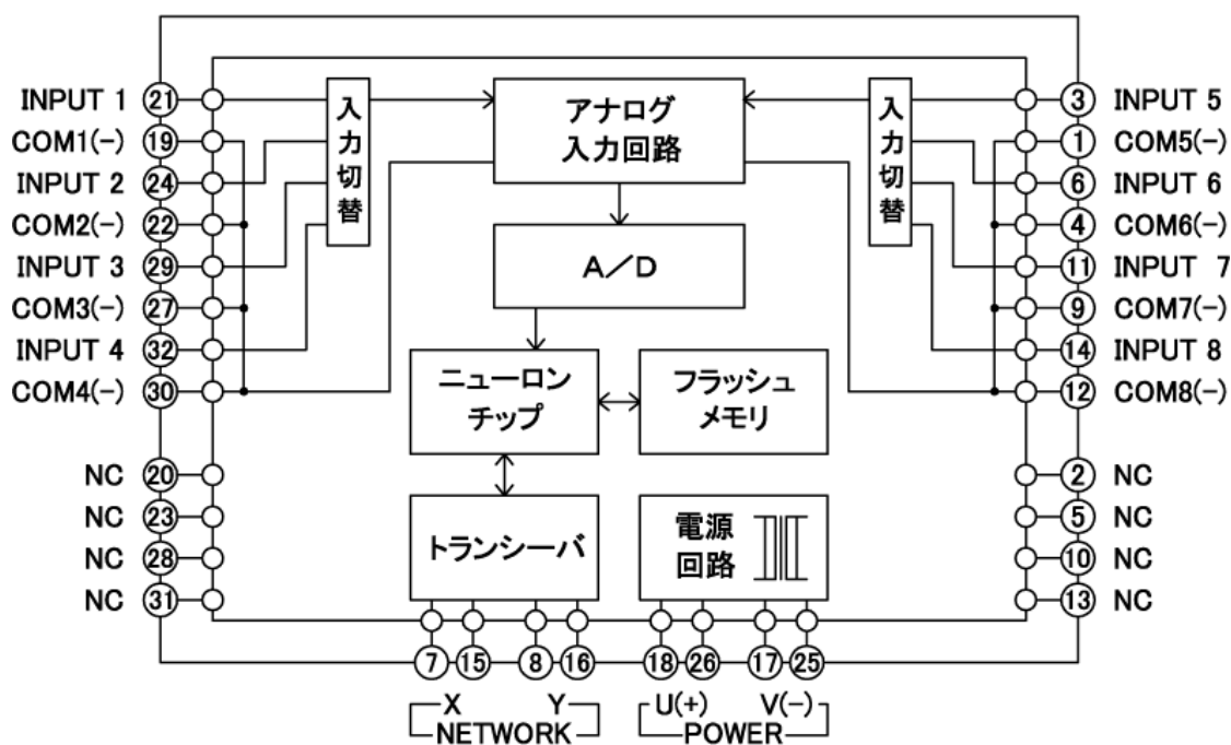
A18F回路ブロック図
