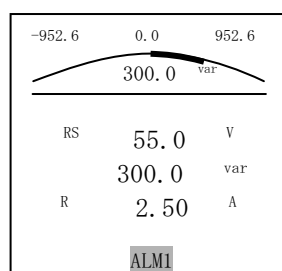
警報 1 警報発生中 [ALM1]点滅
