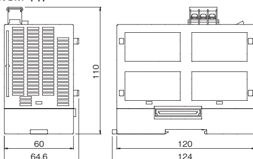
WJM 本体
