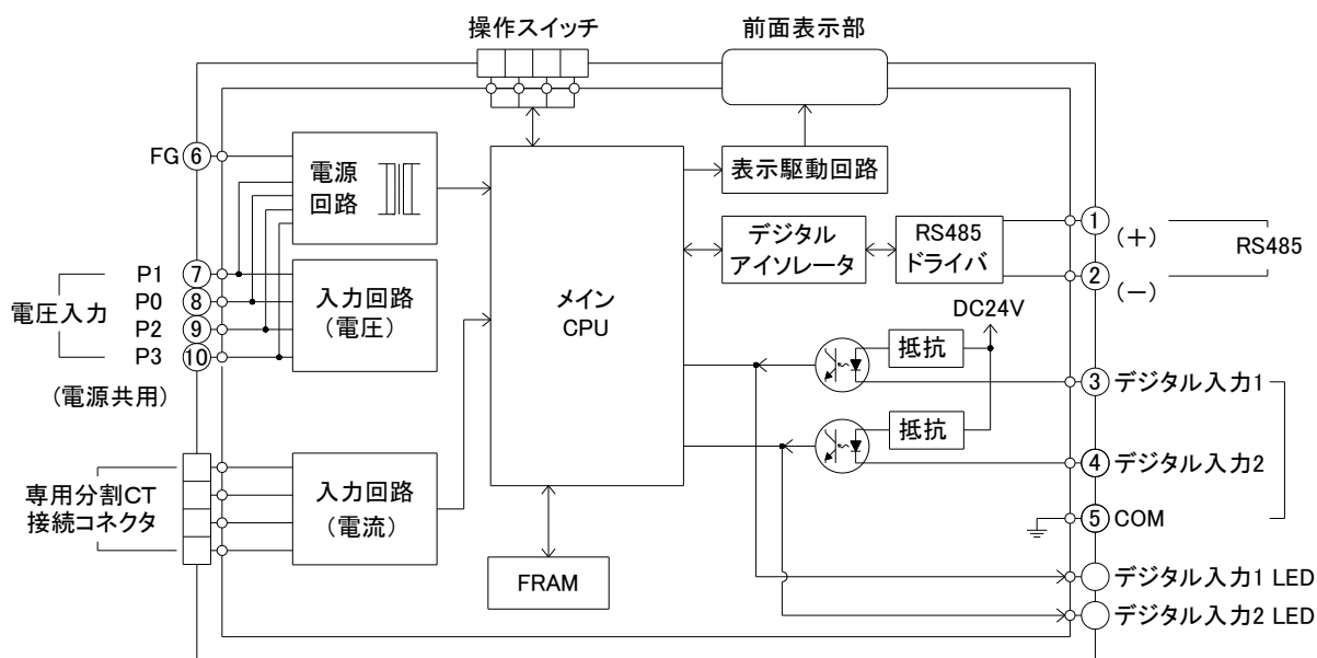
図 8-1 回路ブロック図 WMS-HE2DI
