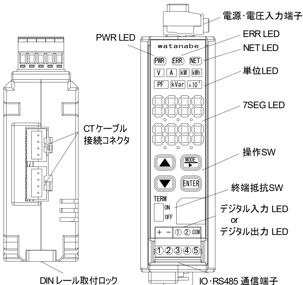
図 5-1 外観説明 WMS-HE2□
