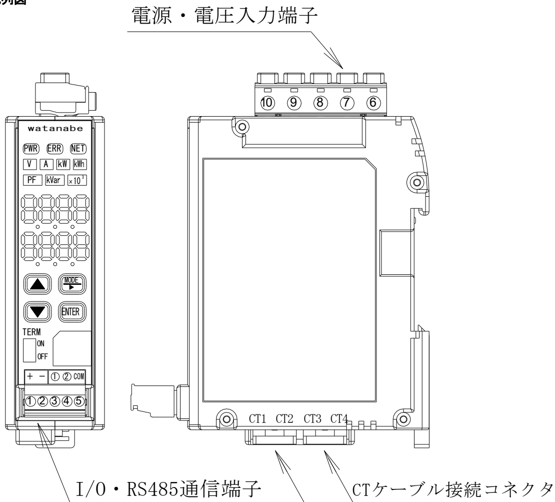
図 7-1 端子配列図 WMS-HE2□
