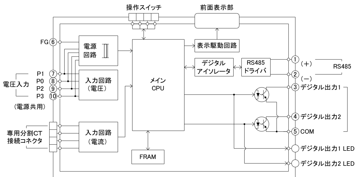
図 8-2 回路ブロック図 WMS-HE2DO
