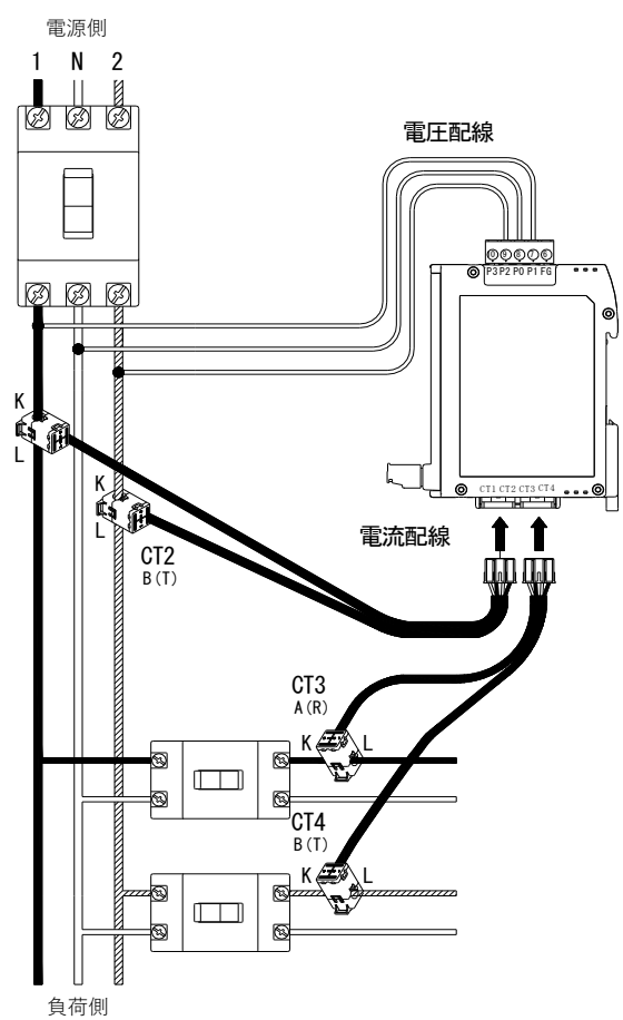
単相3線+単相2線 配線例
