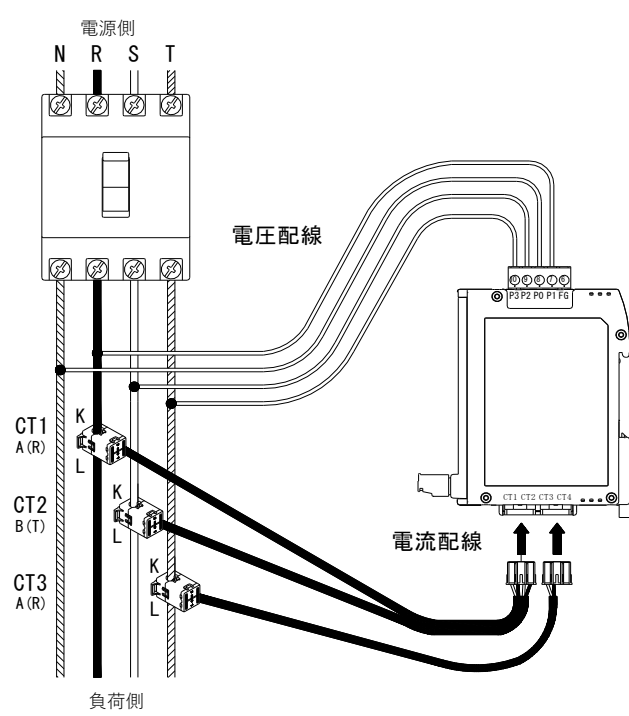
三相4線 配線例
