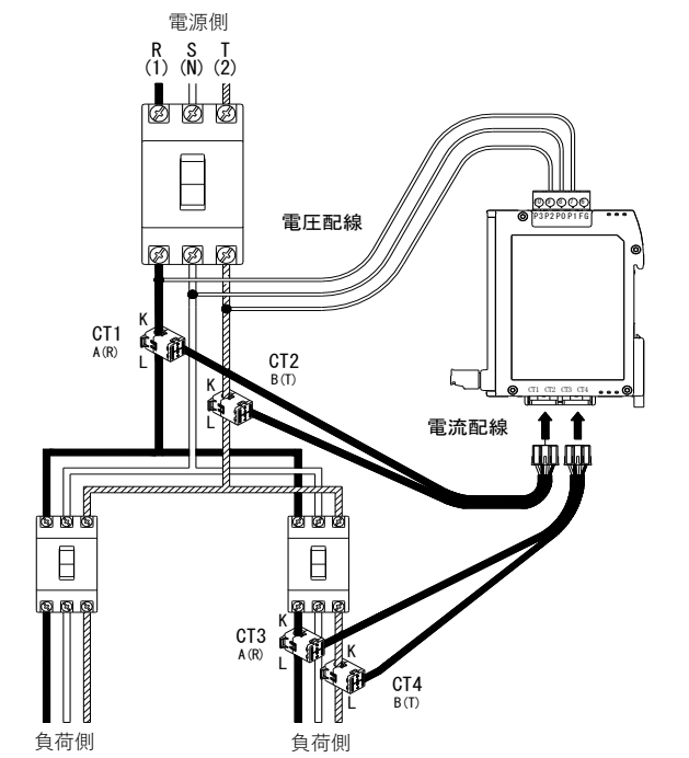
単相3線/三相3線 配線例
