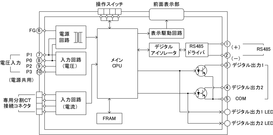
WMS-PE2DI回路ブロック図
