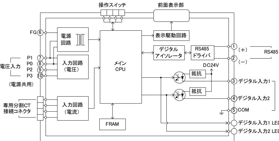
WMS-PE2DI回路ブロック図
