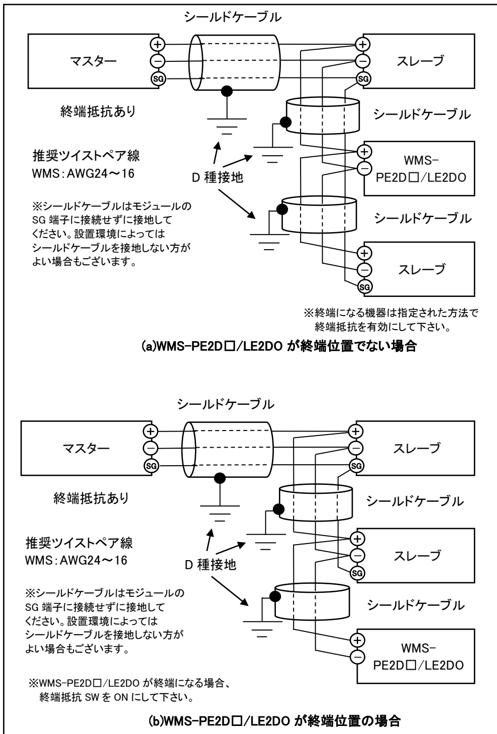
図 2.10 WMS-PE2D□/LE2DOのModbus接続
