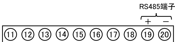
図 2.2 WLDコネクタ
