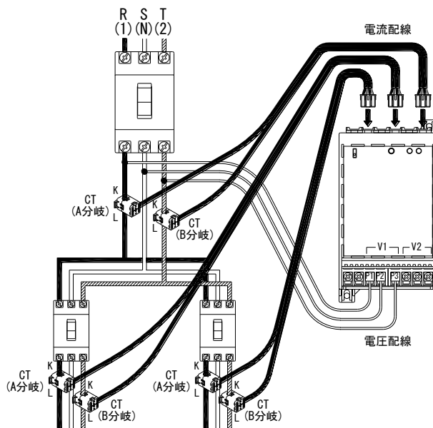
図 4.2 WMS-PE6N配線例
