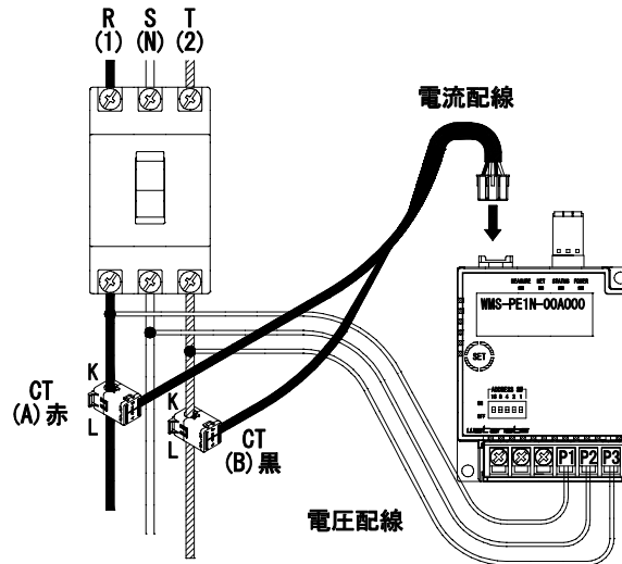
図 4.1 WMS-PE1N配線例
