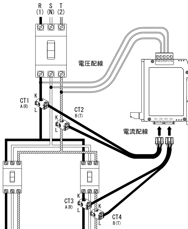
図 4.3 WMS-PE2D□/LE2DO配線例
