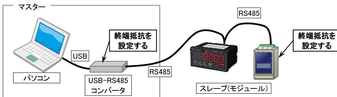
図 2.6 USB-RS485コンバータ使用時の終端抵抗
