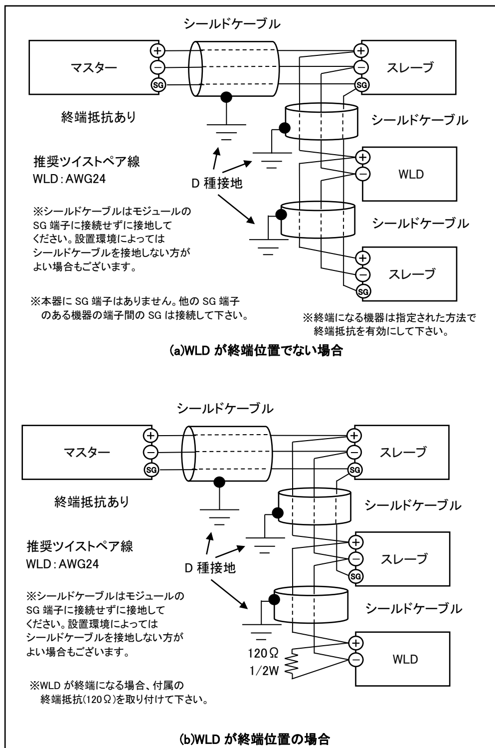
図 2.7 WLDのModbus接続
