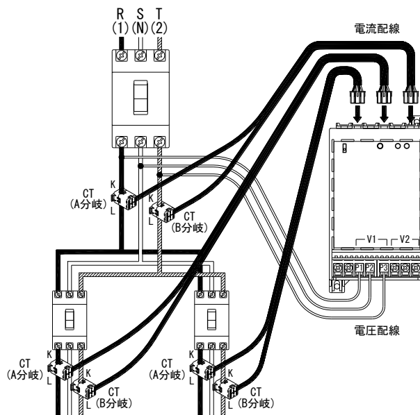
図 4.2 WMS-PE6N配線例
