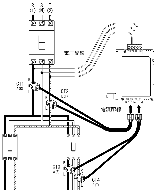
図 4.3 WMS-PE2D□配線例
