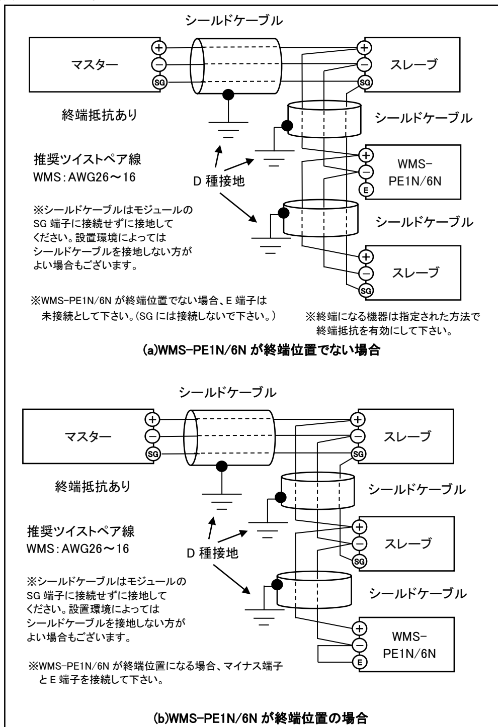
図 2.8 WMS-PE1N/6NのModbus接続
