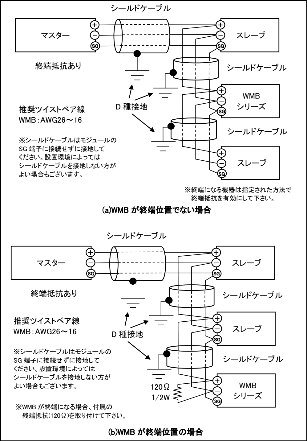
図 2.9 WMBシリーズのModbus接続
