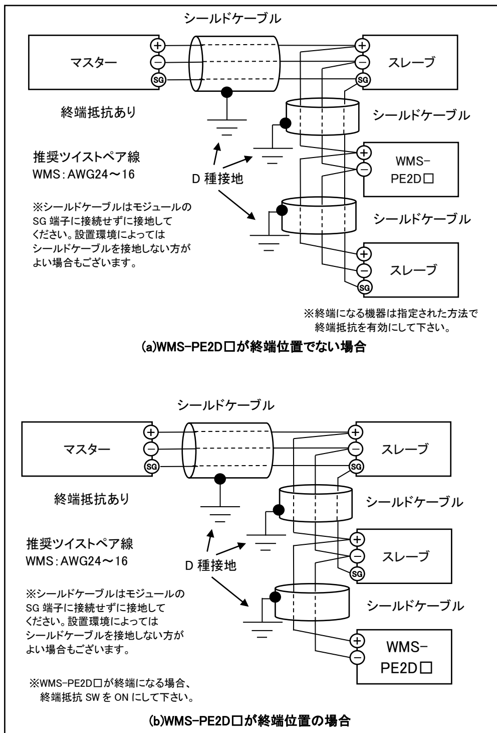
図 2.10 WMS-PE2D□のModbus接続
