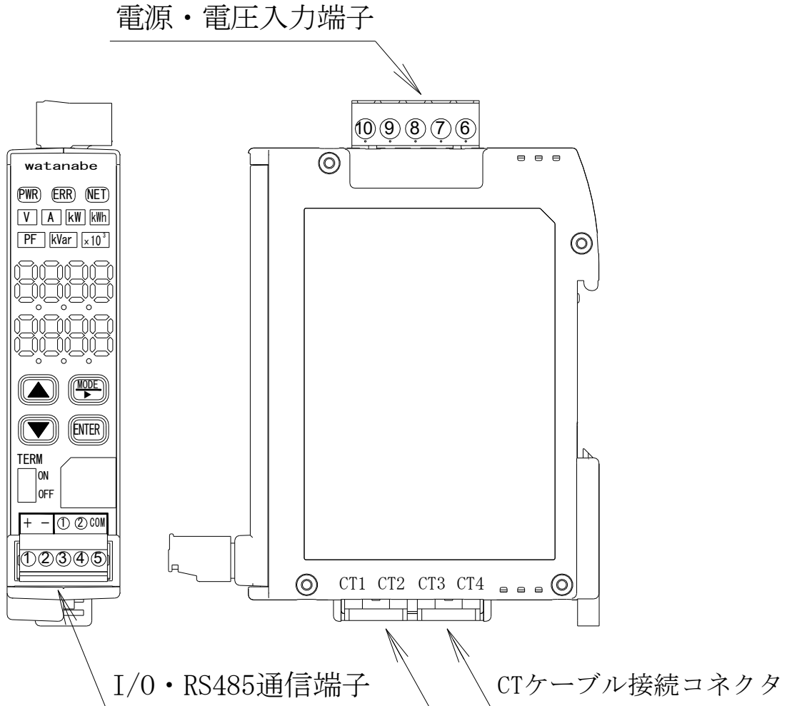
図 7-1 端子配列図 WMS-PE2□
