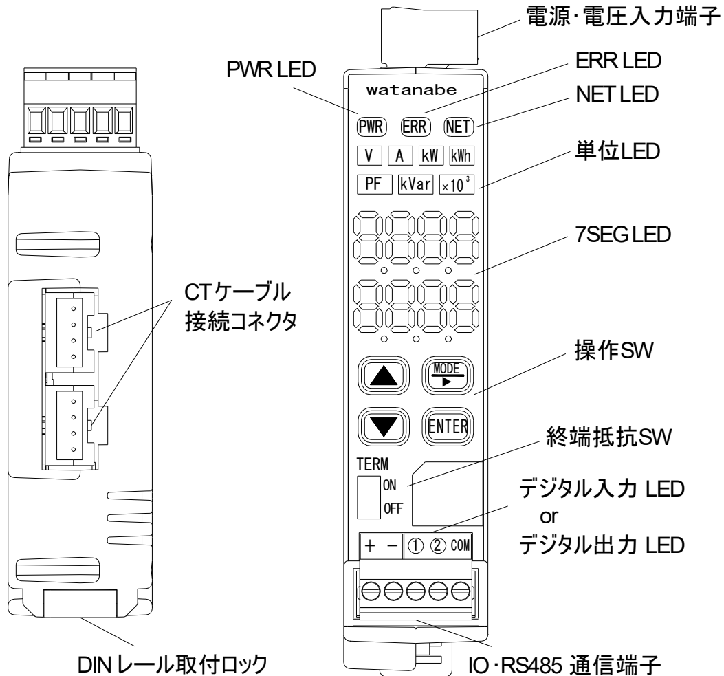
図 5-1 外観説明 WMS-PE2□
