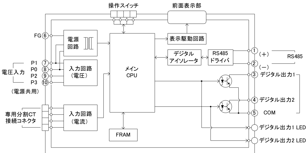
図 8-2 回路ブロック図 WMS-PE2DO/WMS-LE2DO
