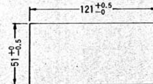
パネル切穴
