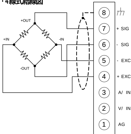
・4線式結線図
