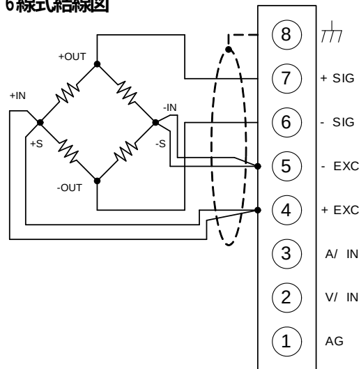
・6線式結線図
