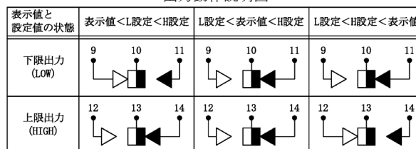
出力動作説明図
