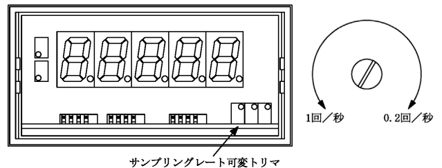
サンプリングレート可変トリマ
