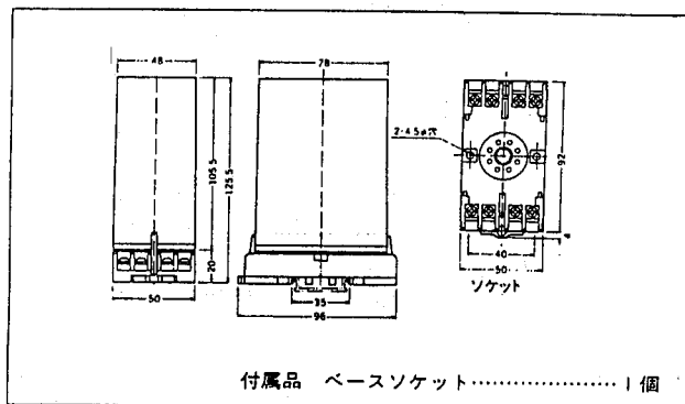
外形寸法図
